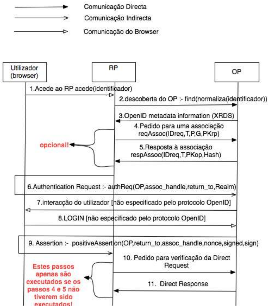
Figura 3.5 mensagens trocadas entre RP e OP sobre o protocolo OPenID
