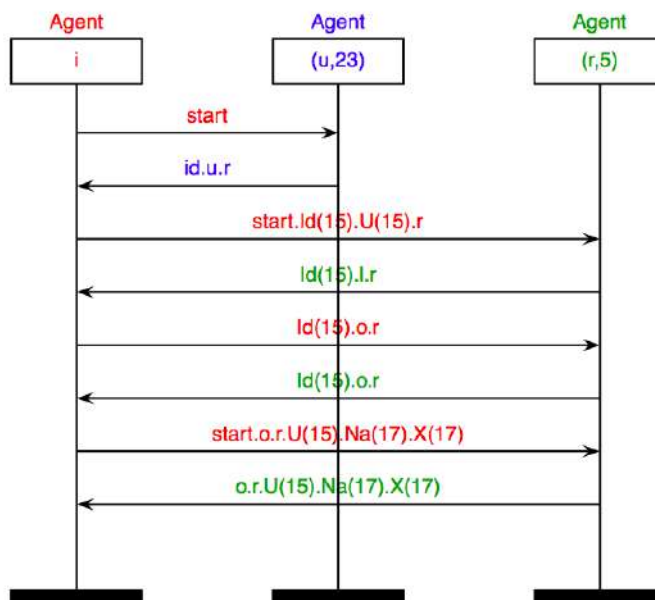
Figura 4.1 Imagem do ataque disponibilizado pela aplicação web do AVISPA para o primeiro cenário
