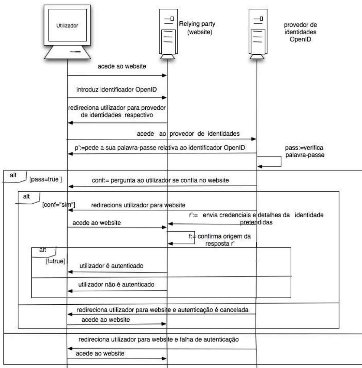
Figura 3.4 Esquema do funcionamento do OPenID segundo a perspectiva do utilizador
