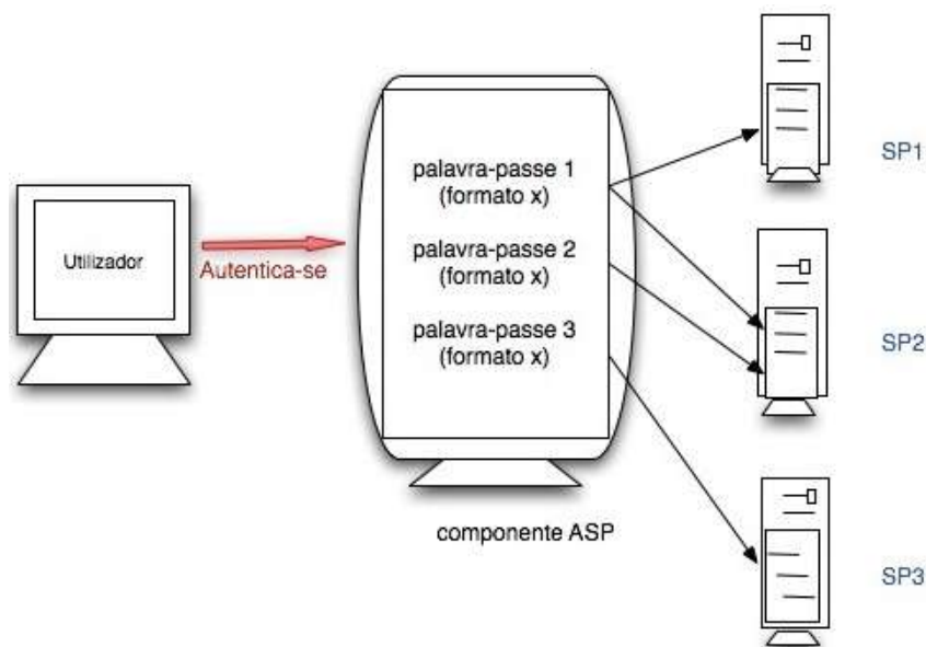
Figura 3.3 Cenário True-SSO
