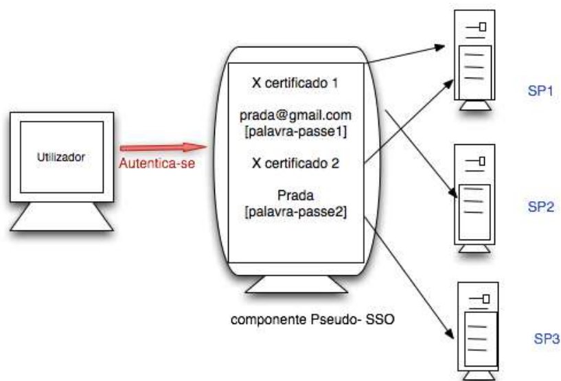
Figura 3.2 Cenário Pseudo-SSO
